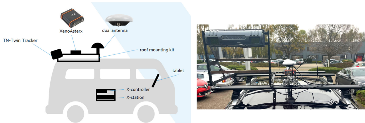
「TN-Twin Tracker」の概要(図左)と実際に車両のルーフに取り付けた様子(図右)
