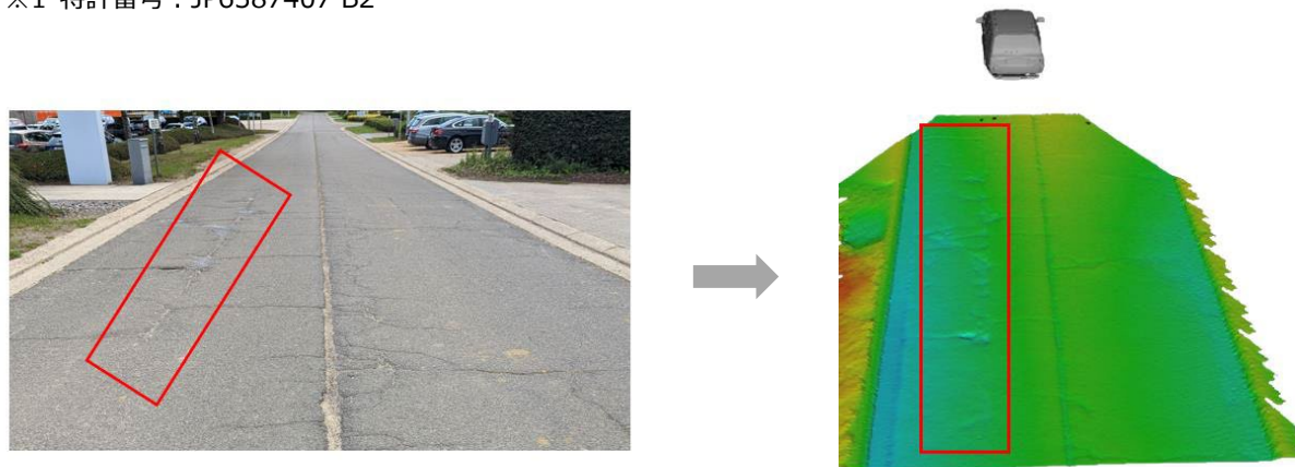
2 車線分の路面凹凸をデジタル化(イメージ)
